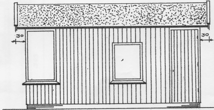
ZIJGEVEL (Z)
